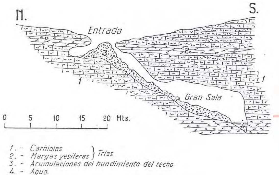
Corte geológico de la Cueva de Montesinos.
